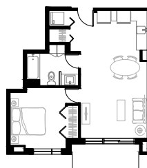
Logement type K - 1cc 53 m 2
