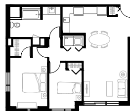
Logement type T - 2cc 78 m 2
