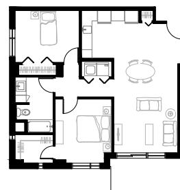
Logement type P - 2cc 83 m 2
